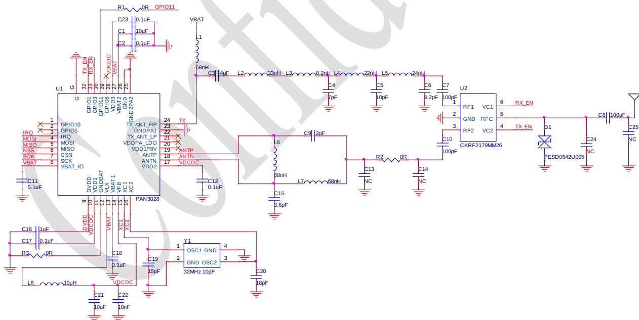
图 6-2 PAN3028 参考原理图（内部 DCDC 供电）
