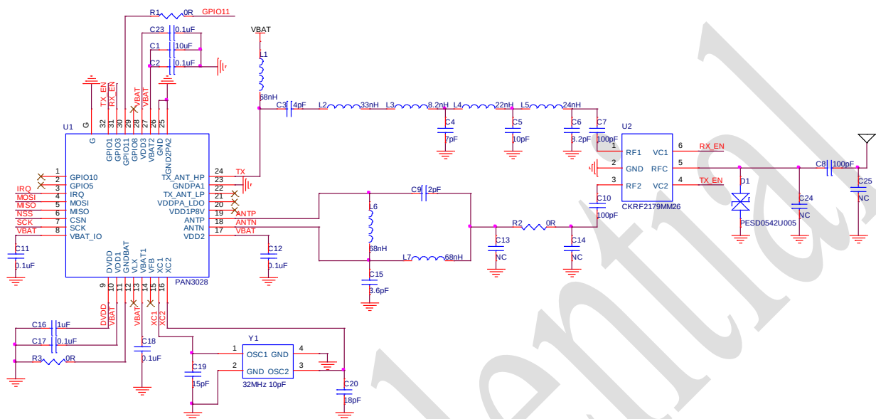
图 6-1 PAN3028 参考原理图（外部 LDO 供电）
