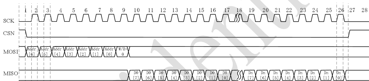
图 7-2 SPI 读时序
