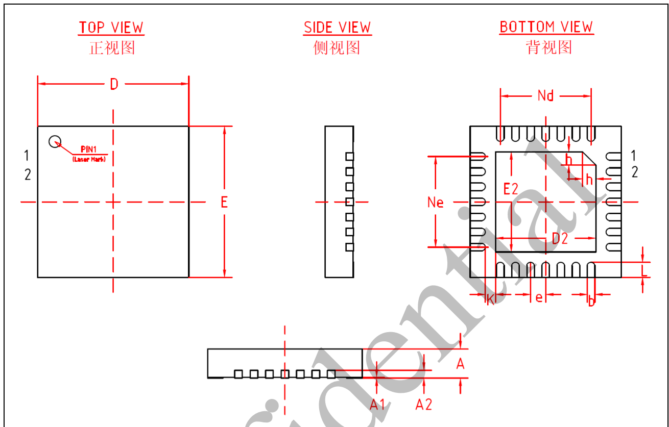
图 14-1 QFN28 封装图
