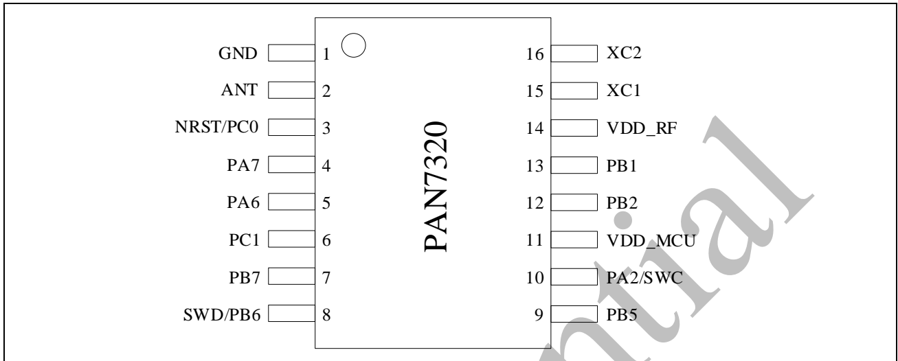
图 4-1 引脚图
