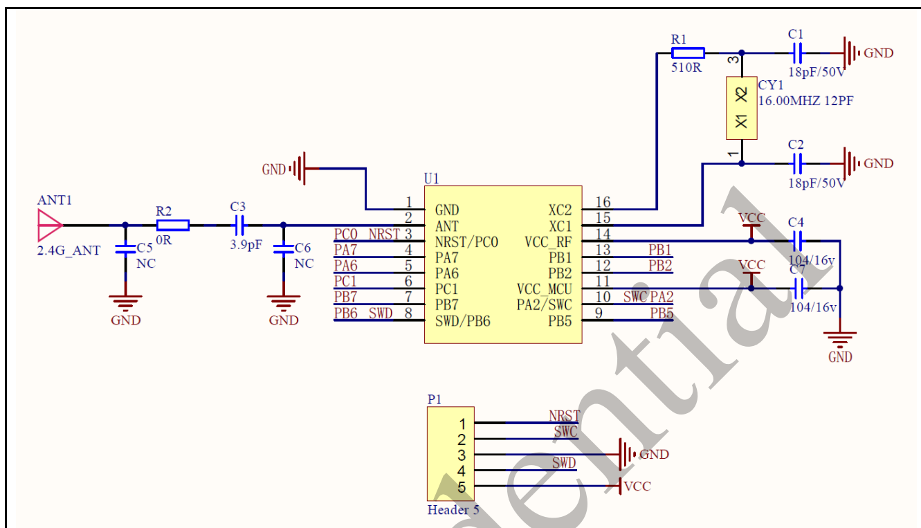
图 5-1 参考原理图
