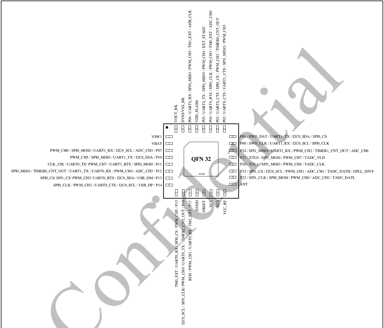
图 4-1 QFN 32 引脚图
