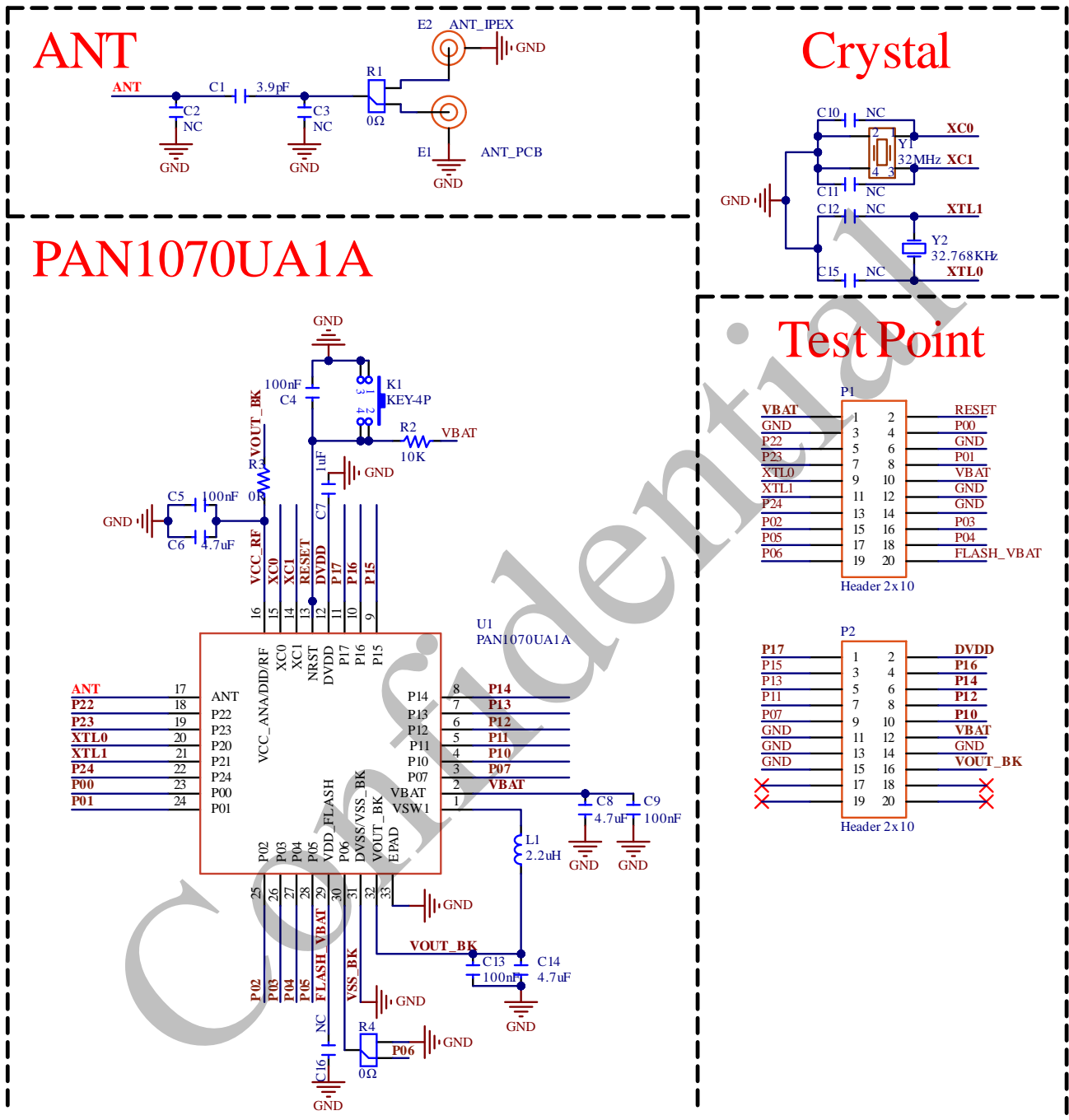
图 6-1 QFN32 参考原理图
