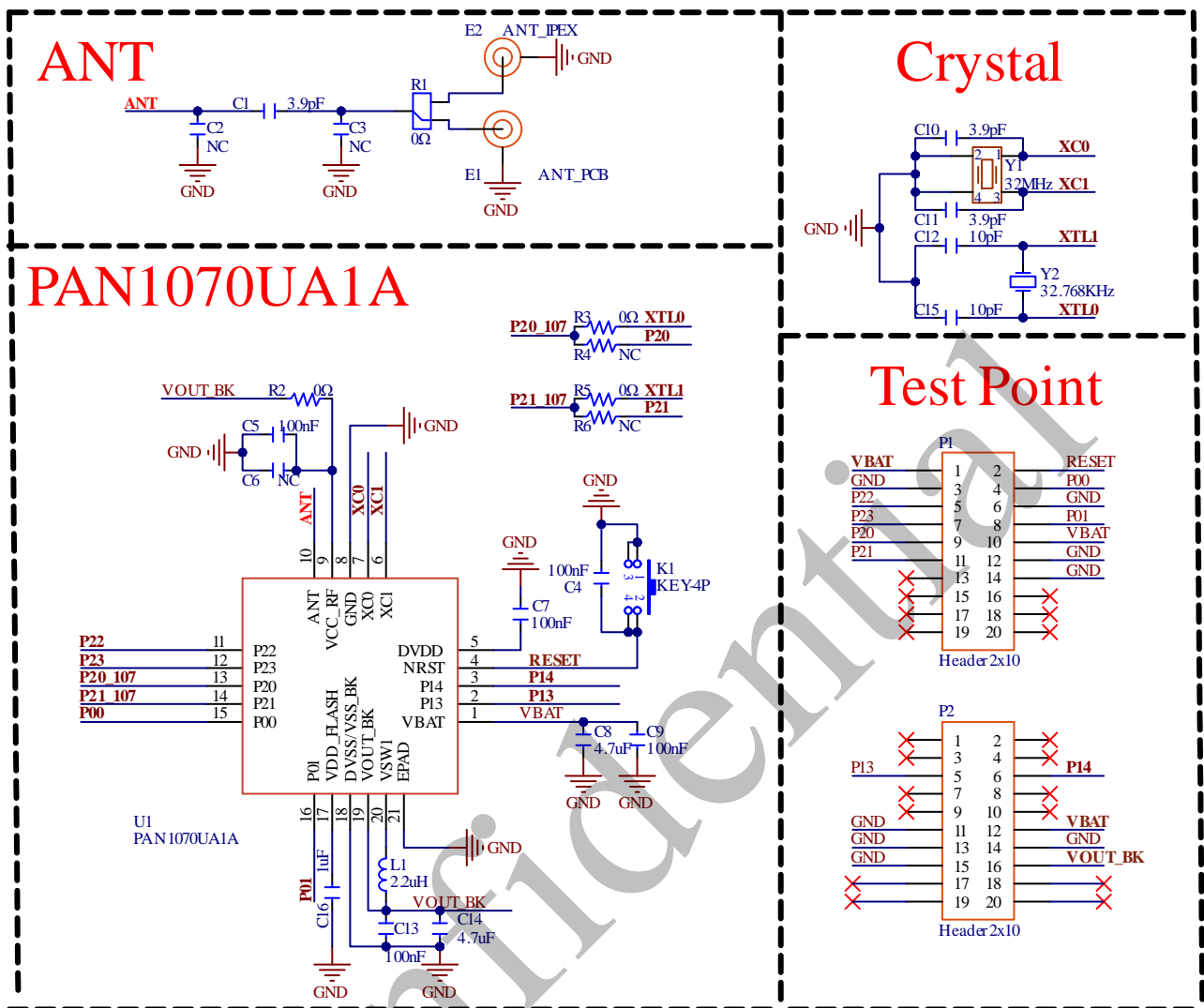
图 6-2 QFN20 参考原理图
