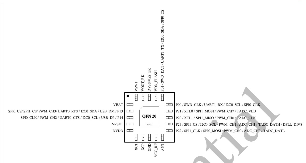
图 4-2 QFN 20 引脚图
