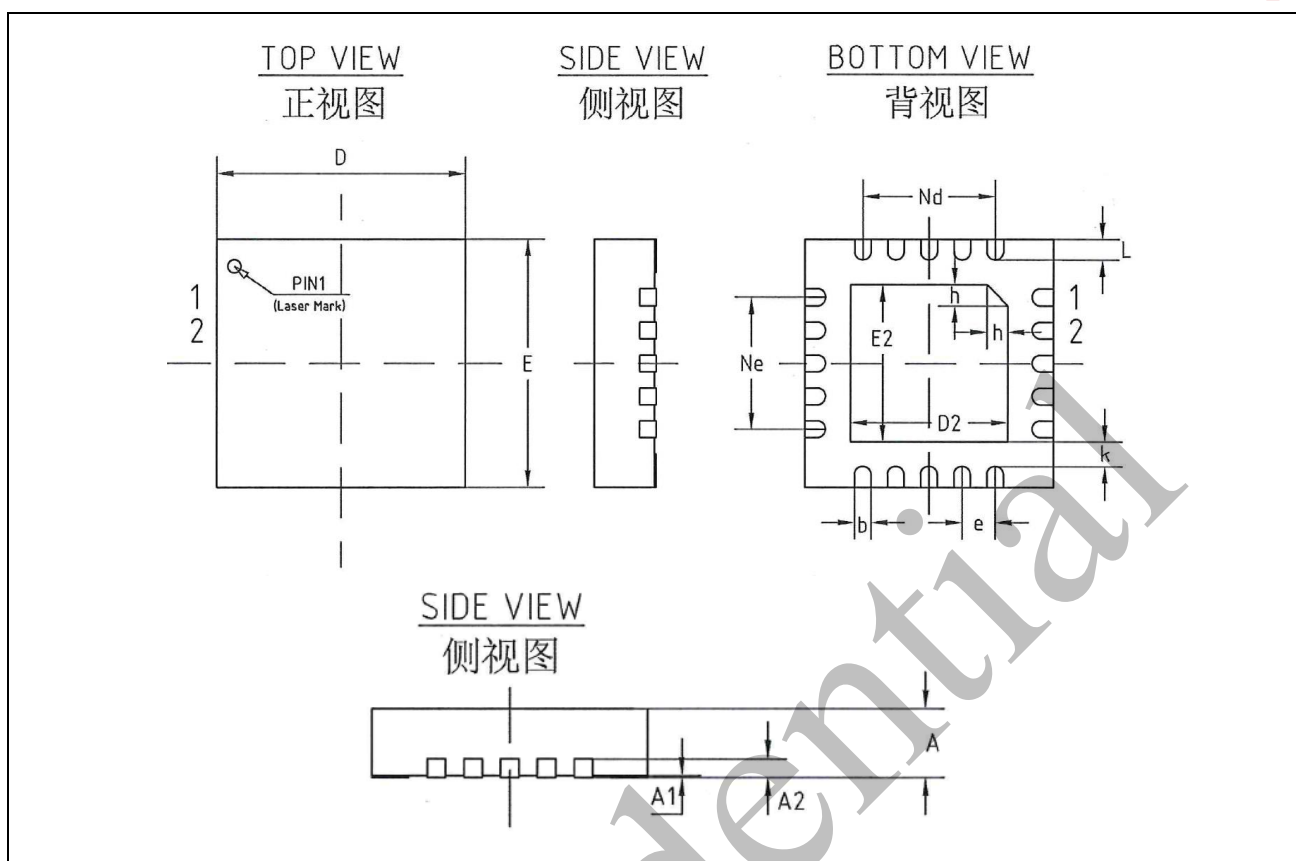
图 7-2 QFN20 封装图
