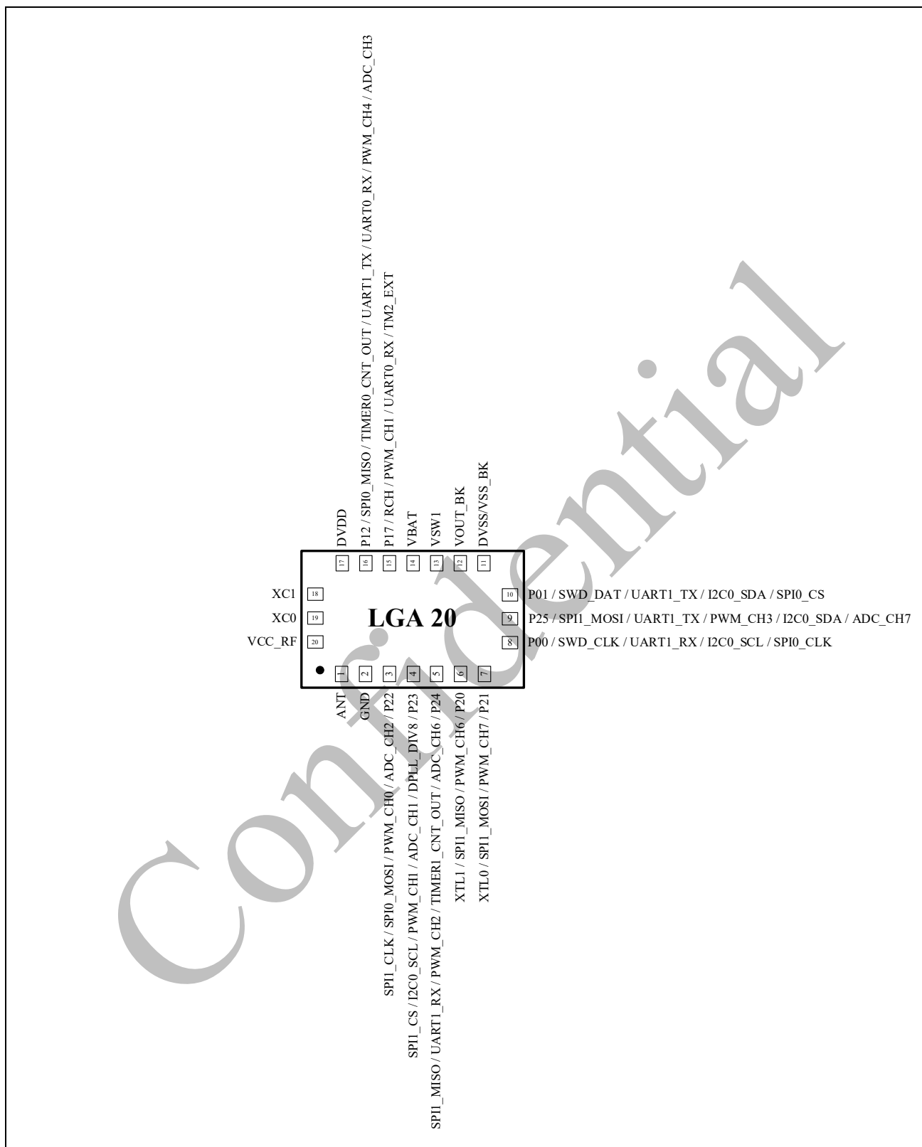
图 4-4 LGA 20 引脚图
