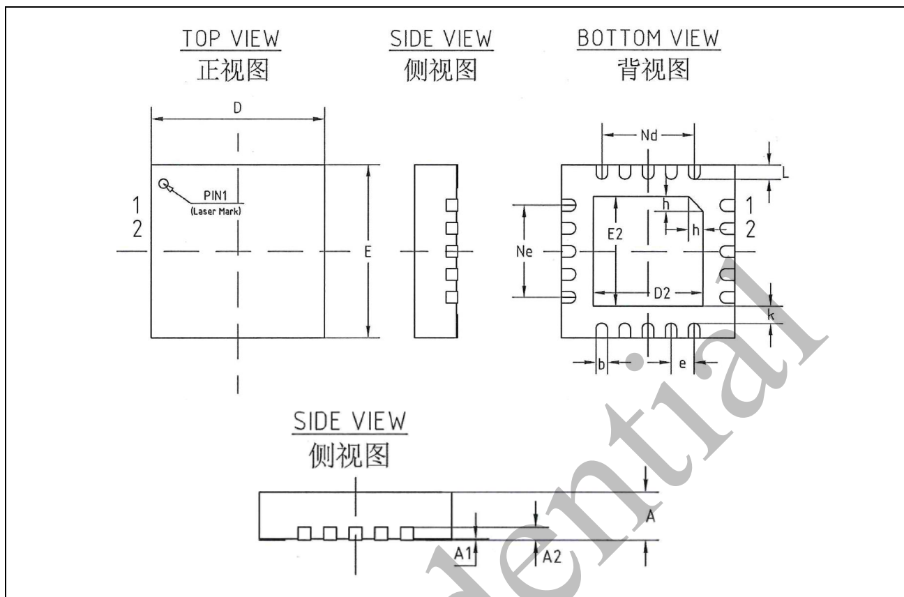
图 7-3 QFN20 封装图
