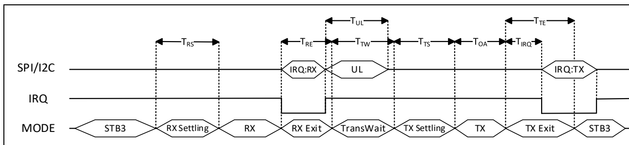
图 6-6 增强型单包接收时序图
