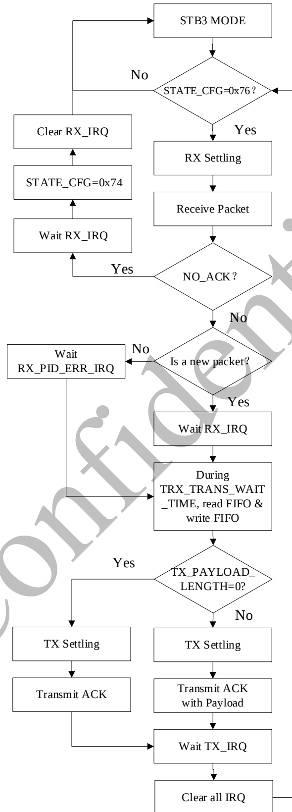
图 8-7 增强模式接收流程图
