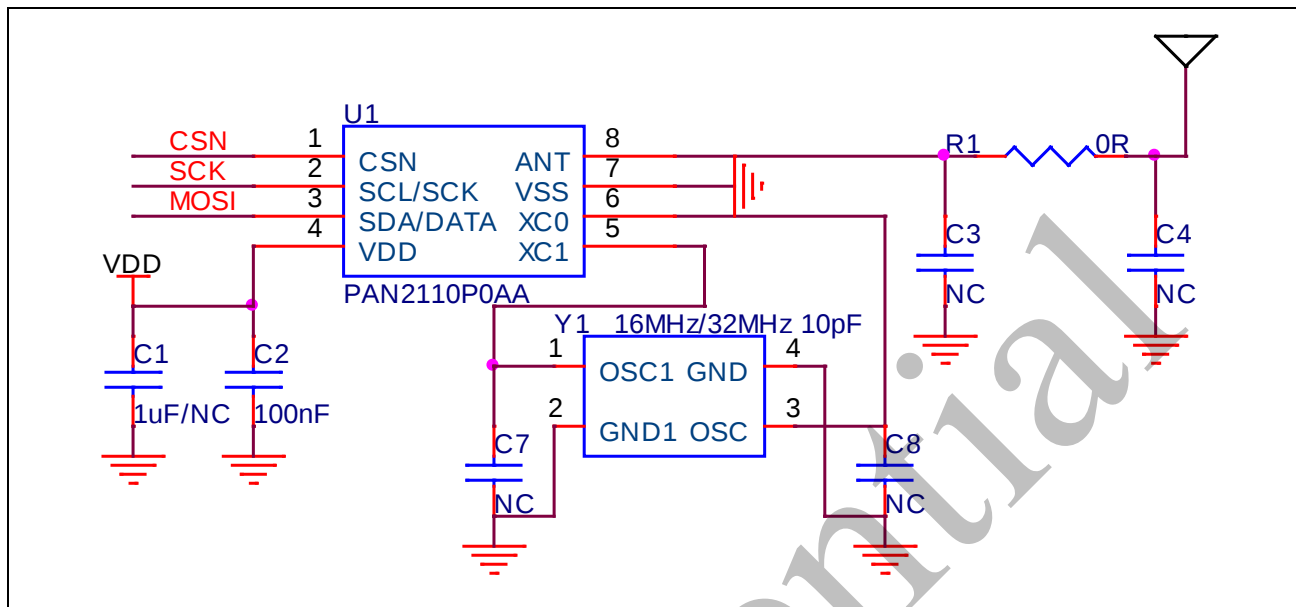
图 11-1 参考原理图
