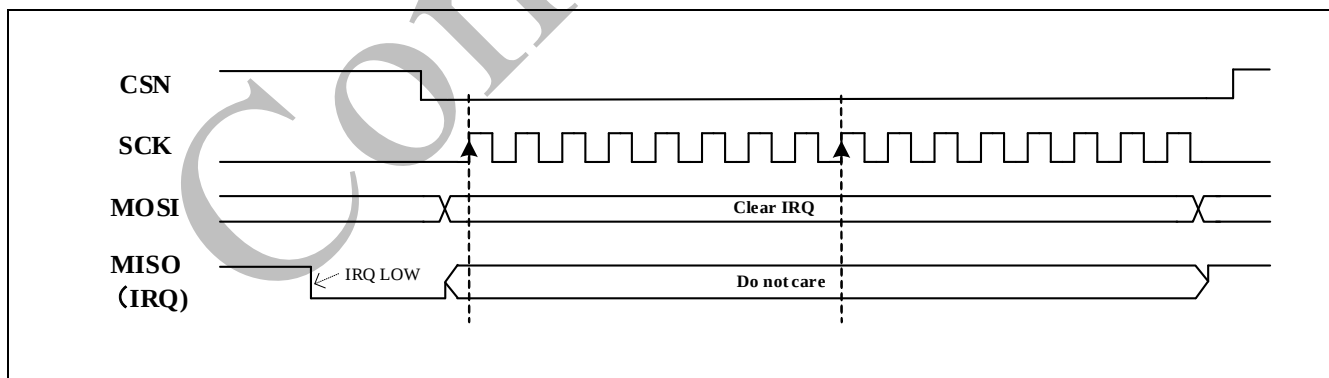
图 9-7 四线 SPI MISO 复用 IRQ 时序
