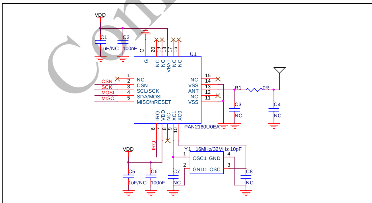
图 11-2 参考原理图
