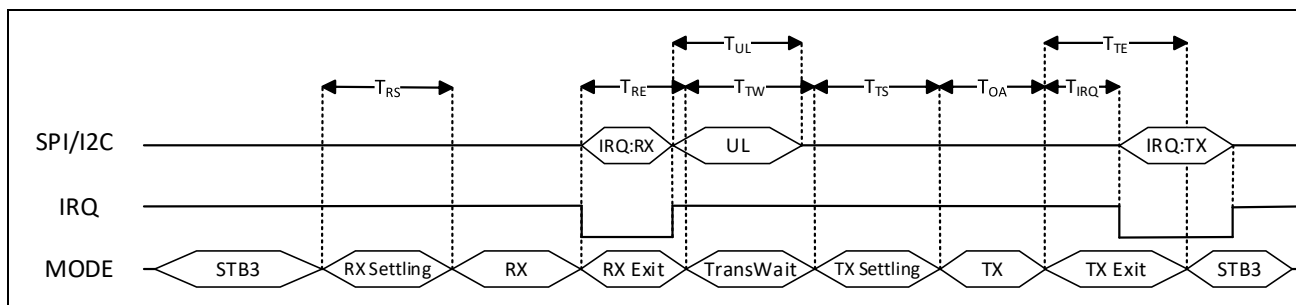
图 6-6 增强型单包接收时序图
