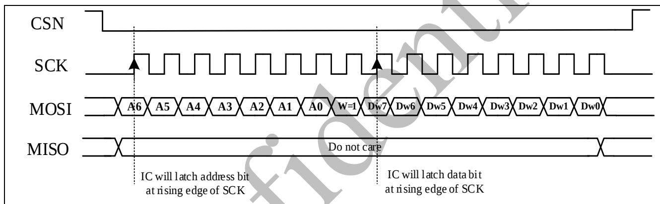
图 9-4 四线 SPI 写时序
