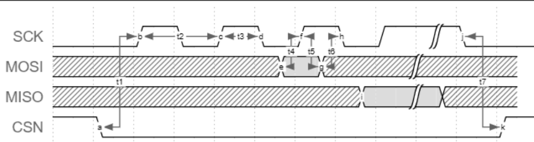
图 7-5 四线 SPI 时序要求图
