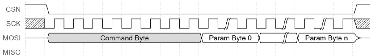
图 7-3 写命令时序
