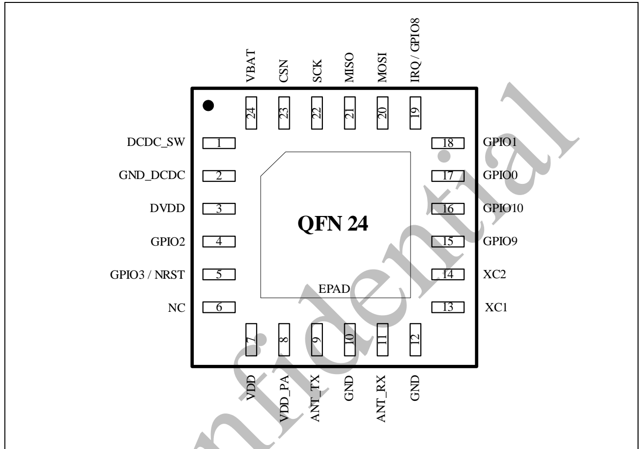
图 4-1 QFN24 引脚图
