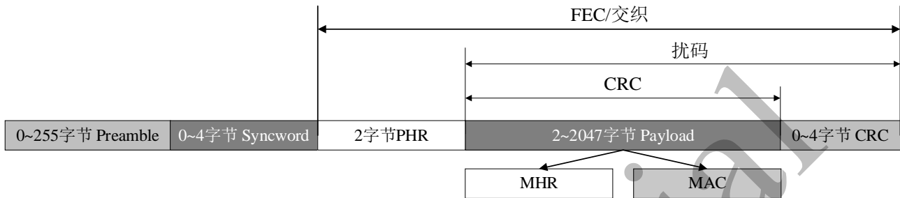
图 9-5 802.15.4g 帧结构
