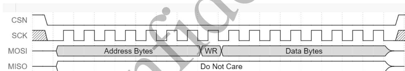
图 7-1 SPI 写特殊寄存器时序
