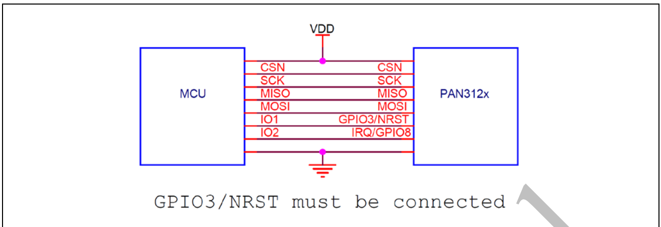
图 11-3 PAN312x 与 MCU 连接应用框图
