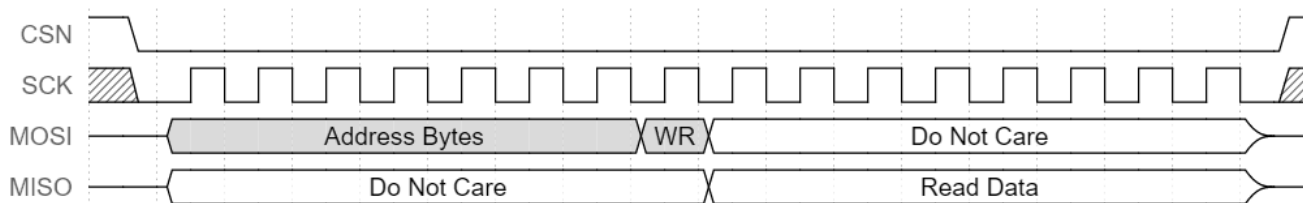
图 7-2 SPI 读特殊寄存器时序
