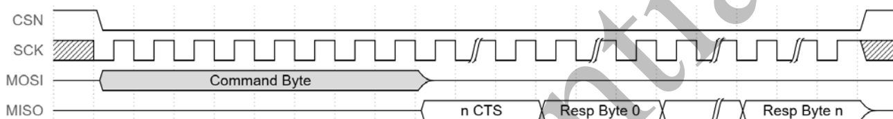
图 7-4 读命令时序
