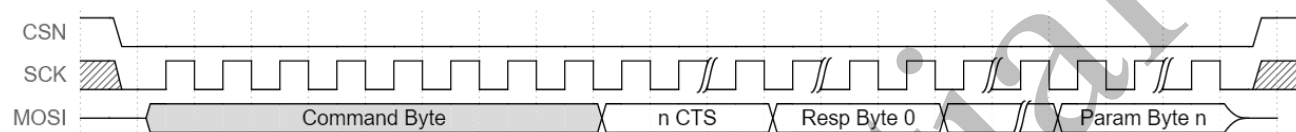
图 7-9 Host 读命令时序
