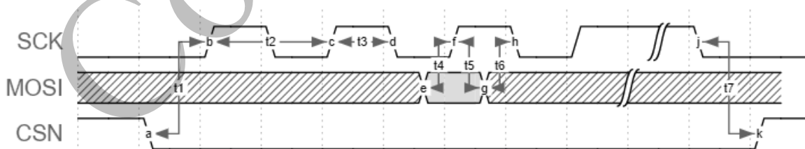
图 7-10 三线 SPI 时序要求图
