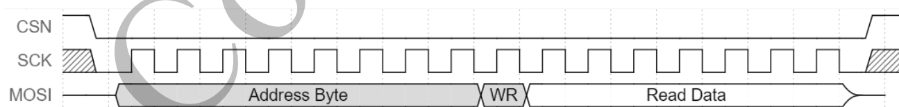
图 7-7 3 线 SPI 读时序
