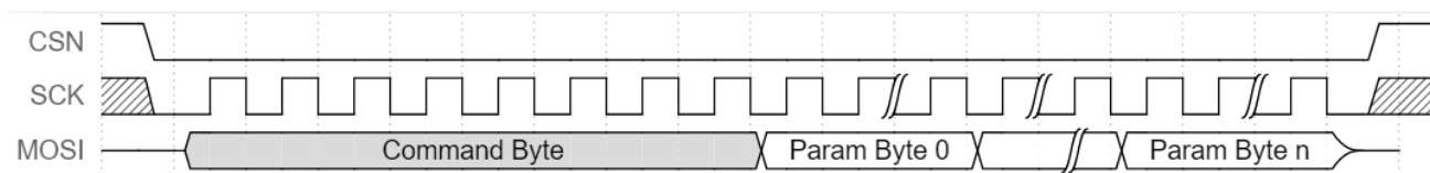
图 7-8 Host 写命令时序
