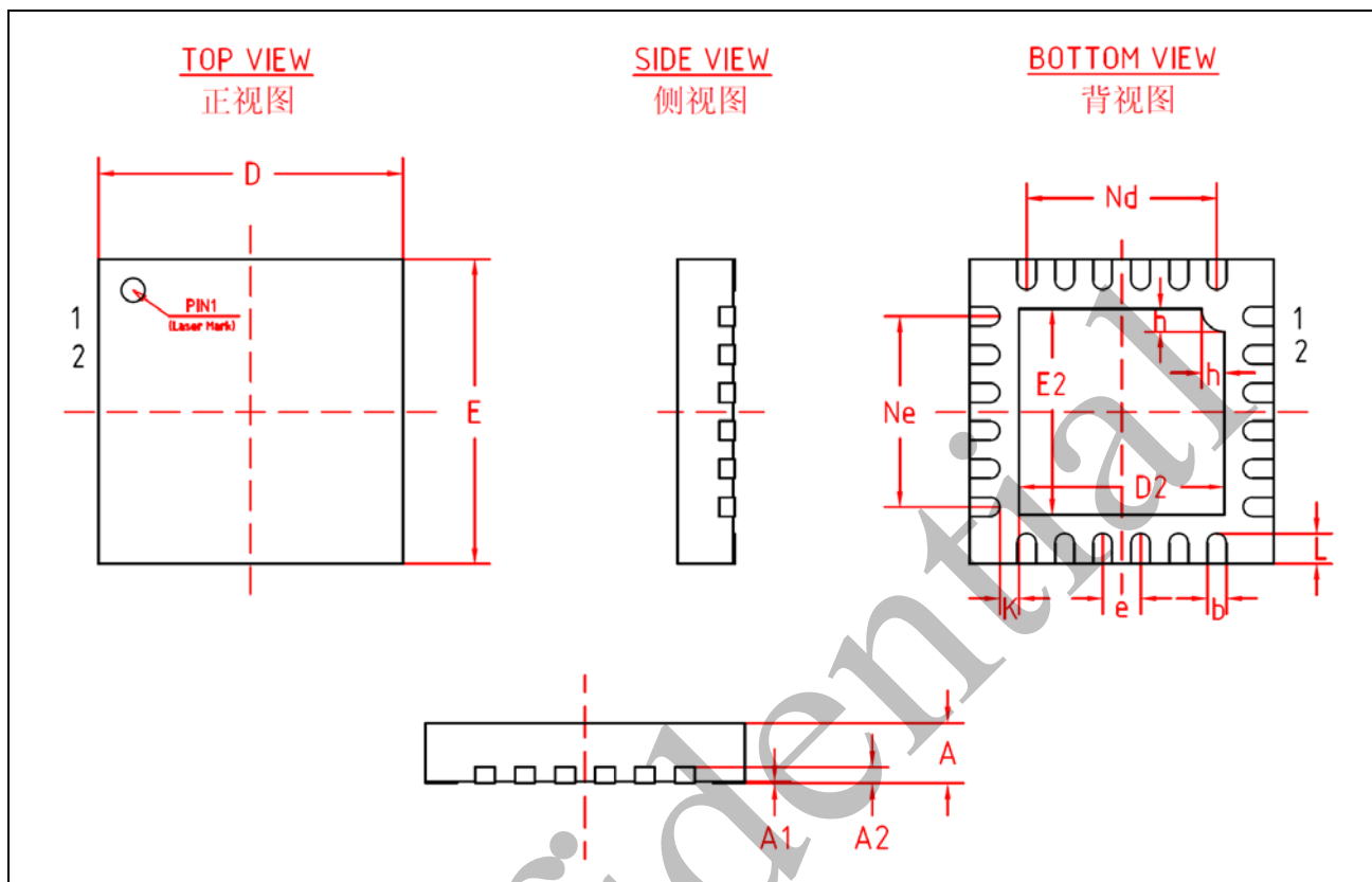
图 12-1 封装图
