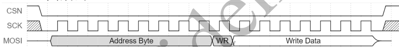
图 7-6 3 线 SPI 写时序
